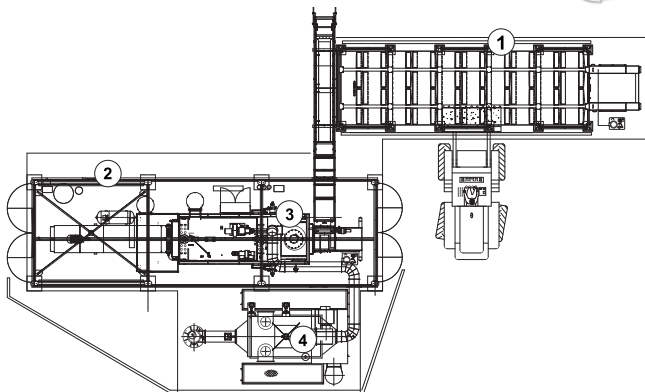
Traitement des fumées Electrofiltre - rejets <20mg/Nm 3
