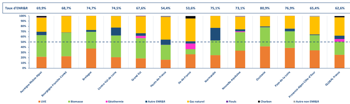
Figure 54 : Bouquet énergétique entrant des réseaux de chaleur par région
