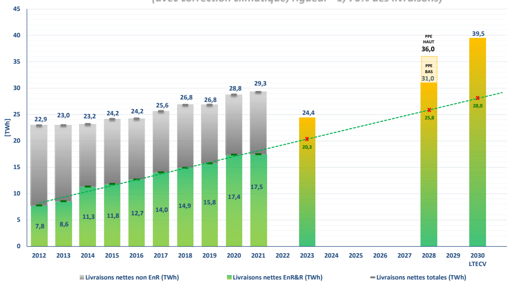
Figure 35 : Rythme prévisionnel des livraisons d'EnR&R corrigées du facteur climatique
