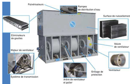
Figure 60 : Tour ouverte - principe et équipement
