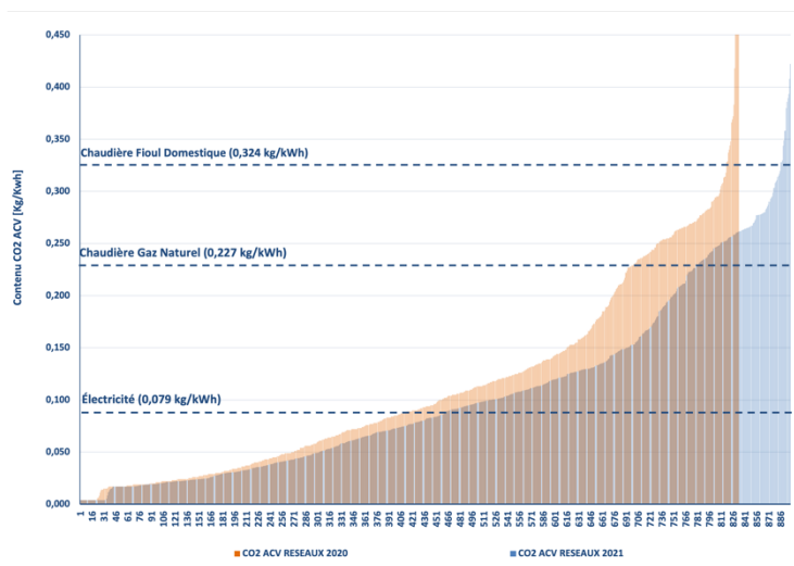
Figure 24 : Dispersion des réseaux de chaleur en termes d'émissions de CO 2 en ACV
