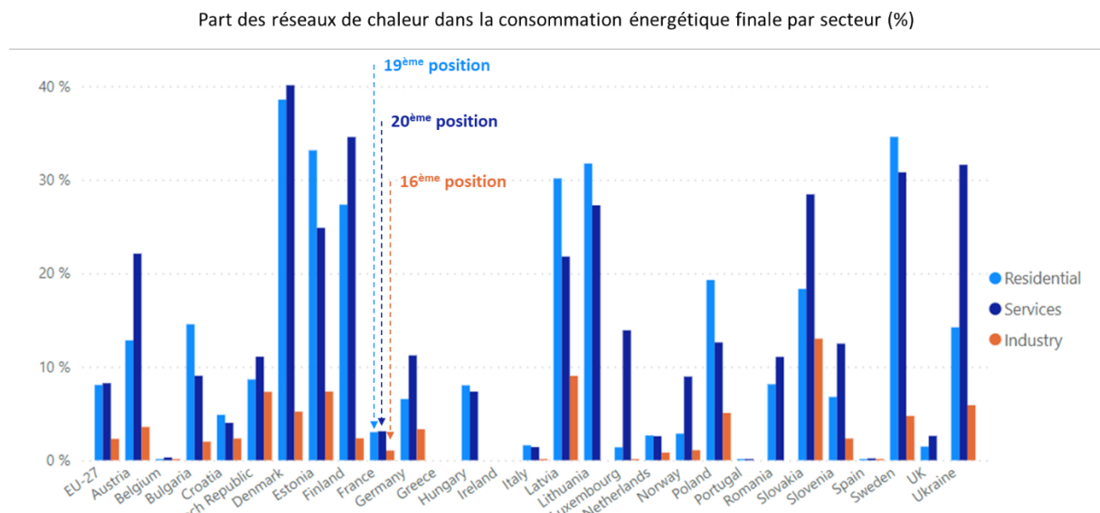
Figure 4 : Comparatif de la couverture des besoins en chaleur par secteurs (%).
