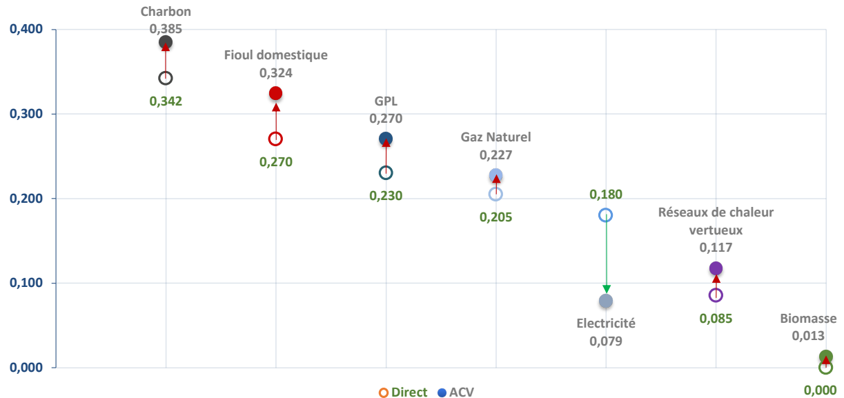
Figure 45 : Comparisons des contenus carbone des énergies selon les méthodologies RT2012 et RE2020
