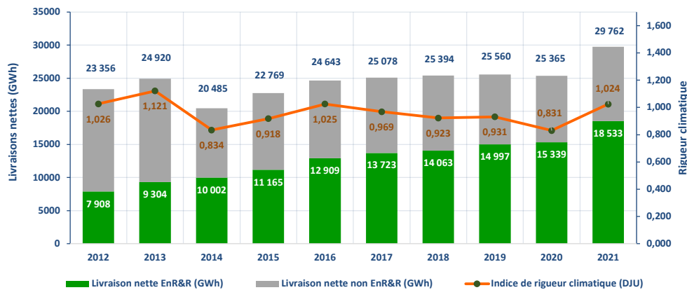
Figure 39 : Évolution des livraisons aux utilisateurs entre 2012 et 2021
