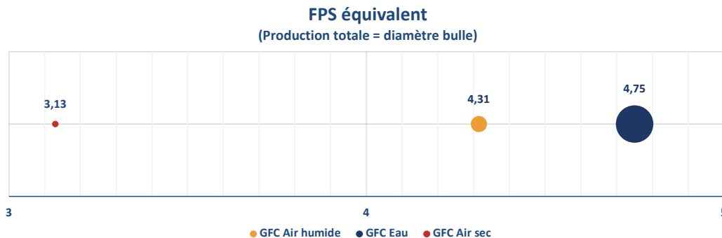
Figure 67 : Facteur de performance saisonnier (FPS) des groupes froids à compression par type de source renouvelable
