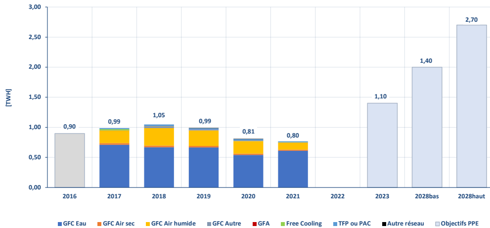
Figure 71 : Objectif de développement des réseaux de froid
