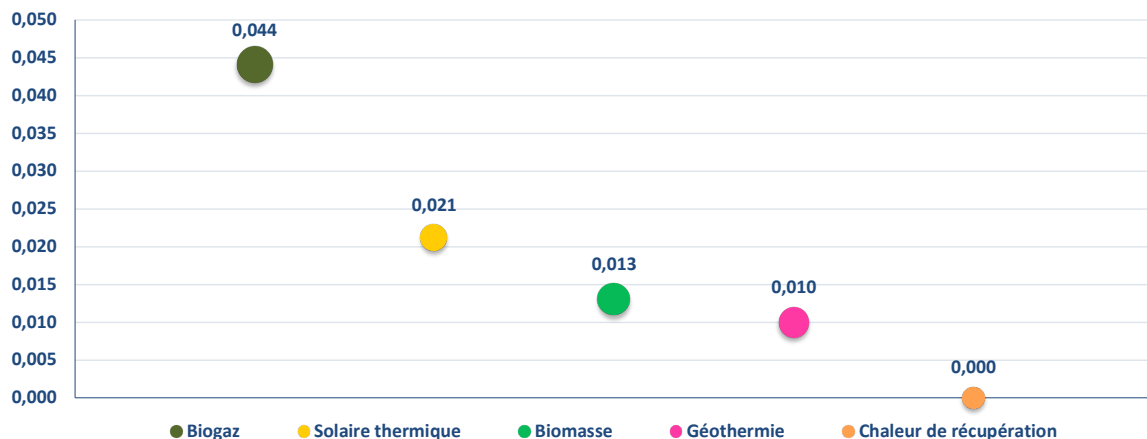
Figure 27 : Contenus en CO 2 des sources d'énergie renouvelable et de récupération
