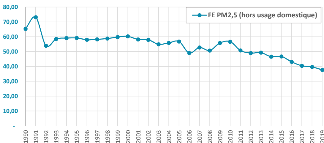
Facteurs d'émission de PM_{2,5} du Bois-énergie (en g/GJ)
