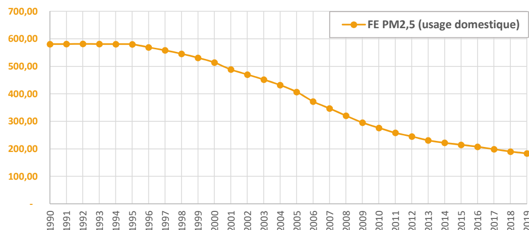
Facteurs d'émission de PM_{2,5} du Bois-énergie (en g/GJ)
